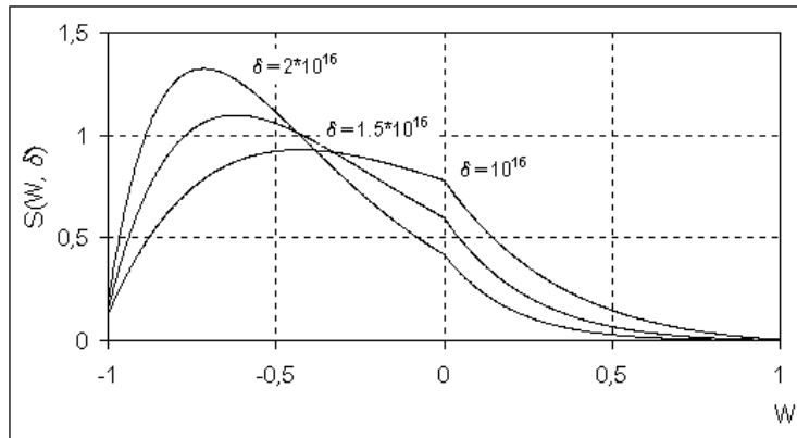
Рис. 3. Энергетический спектр образованных протонов S(W, \delta) для различных толщин мишени \delta .
