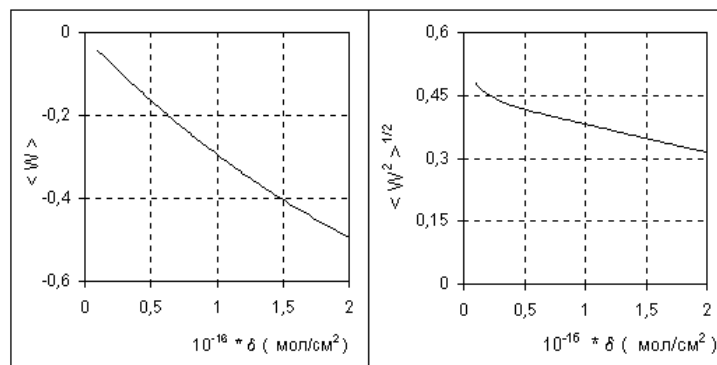
Рис. 4. Зависимость среднего изменения энергии протонов \langle W \rangle и среднеквадратичного разброса энергии протонов \langle W^2 \rangle^{\frac{1}{2}} от толщины мишени \delta .
