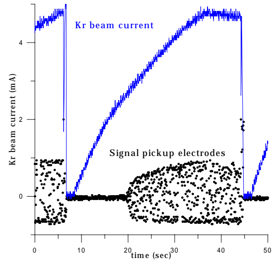
Рис. 2: Сигнал ионного тока и сигнал с пикап-электрода при накоплении ионного пучка на установке SIS (Дармштадт, ФРГ). Энергия ионов 11 МэВ/н, ток электронов 0.5 А.
