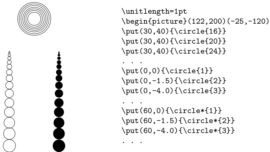
Рис. 11: Полный набор окружностей и кругов для построения рисунков в командных скобках picture .
