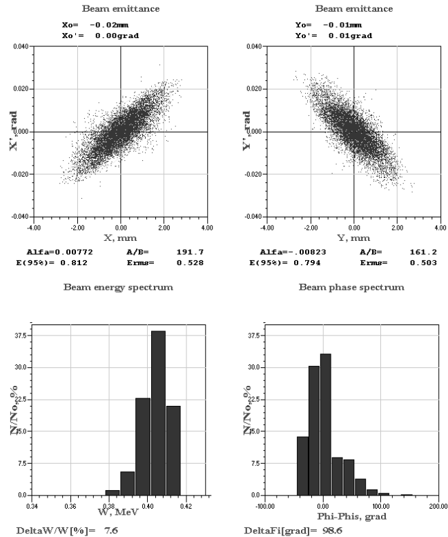
Рис. 4. Пучок на выходе НЧУ, I = 5 мА.
