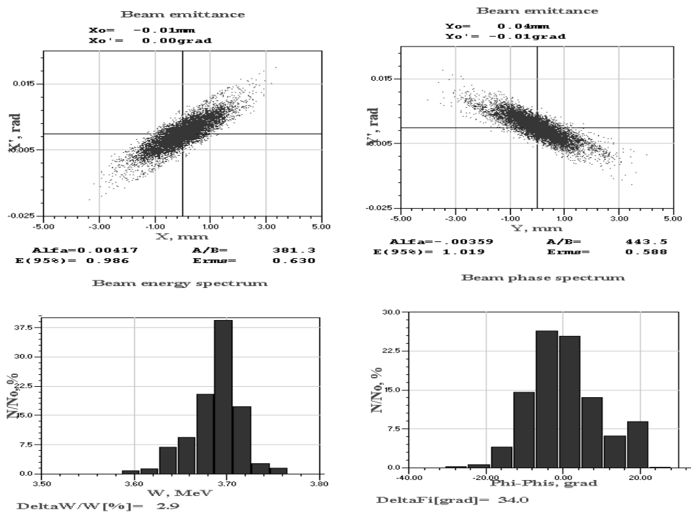
Рис. 7. Пучок на выходе ускорителя, I = 5 мА.
