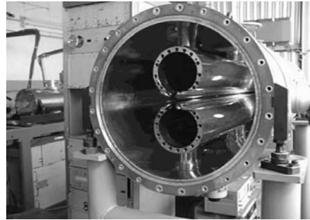
Рис. 2. Поперечное сечение 2N-резонатора.
