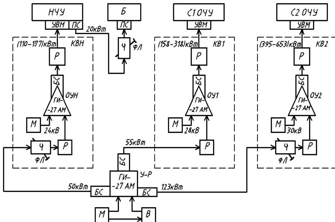
Рис. 8. Структурная схема системы ВЧ-питания. Б – банчер; БС – блок связи ВЧ-усилителя с выходным фидером; В – возбудитель; КВН – канал возбуждения НЧУ; КВ1 – канал возбуждения С1 ОЧУ; КВ2 – канал возбуждения С2 ОЧУ; М – модулятор анодных напряжений; НЧУ – начальная часть ускорителя; ОУН – окончательный усилитель канала КВН; ОУ1 – окончательный усилитель канала КВ1; ОУ2 – окончательный усилитель канала КВ2; ПС – петля связи; Р – рефлектомер; С1 ОЧУ – первая секция ОЧУ; С2 ОЧУ – вторая секция ОЧУ; УВМ – узел ввода мощности; ФЛ – фазосдвигающая линия; У-Р – усилитель-разветвитель.
